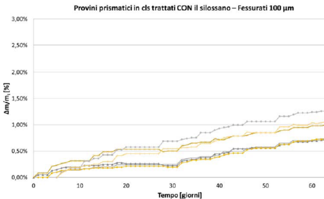
Figura 7: variazione % in peso – provini fessurati a 100 \mu\text{m} trattati con PROTECH
