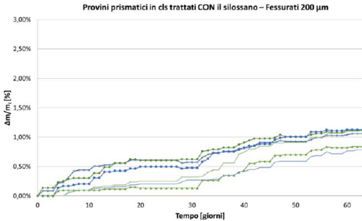
Figura 9: variazione % in peso – provini fessurati a 200 \mu\text{m} trattati con PROTECH
