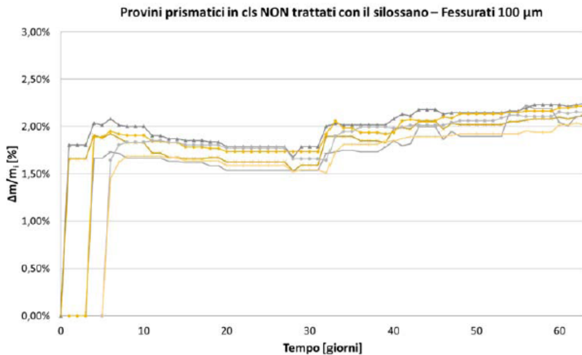
Figura 6: variazione % in peso – provini non trattati fessurati a 100 \mu\text{m}
