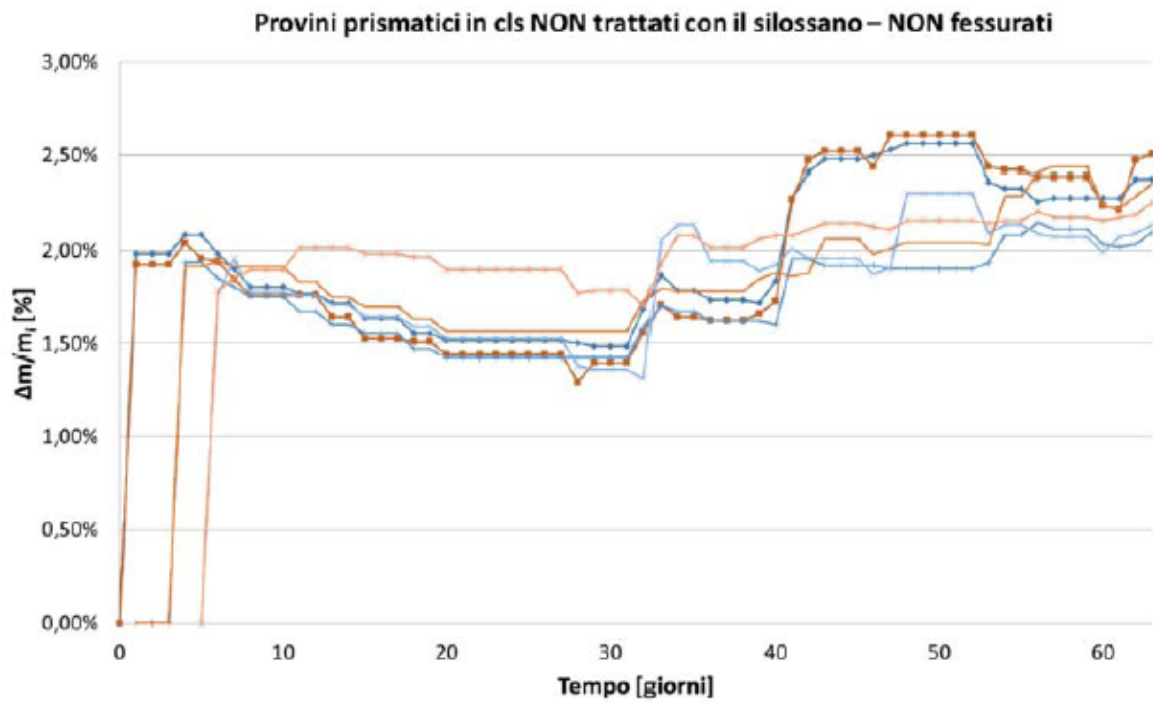
Figura 4: variazione % in peso – provini non trattati non fessurati
