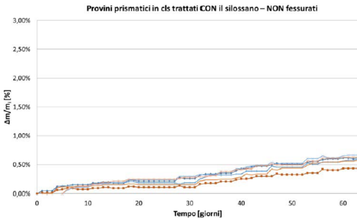
Figura 5: variazione % in peso – provini non fessurati trattati con PROTECH BALCONY
