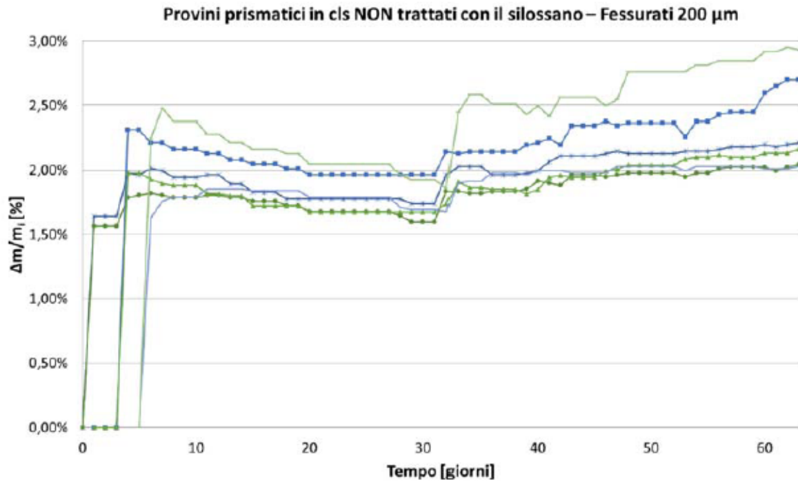
Figura 8: variazione % in peso – provini non trattati fessurati a 200 \mu\text{m}
