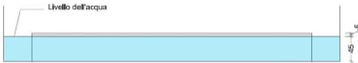
Figura 3: schema della prova per assorbimento d'acqua alla pressione atmosferica.
